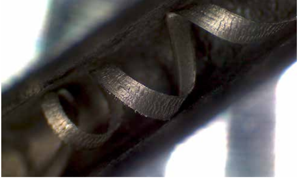
Spiralförmiger Klemmspan.
